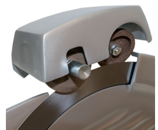
aufgesetzter Schleifparat
